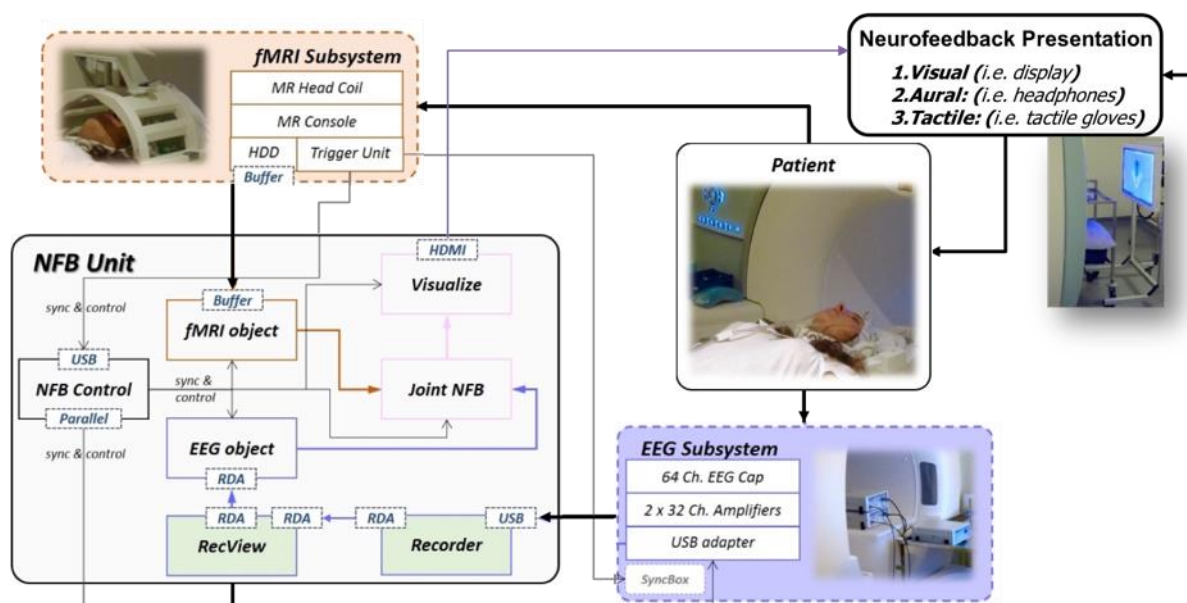
Plateforme multimodale d'enregistrement des signaux EEG et IRM simultanés pour leur traitement en temps-réel
