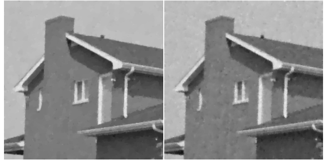
(d) TV recovery. PSNR = 31.44dB. (e) TV OP recovery. PSNR = 30.6dB.
